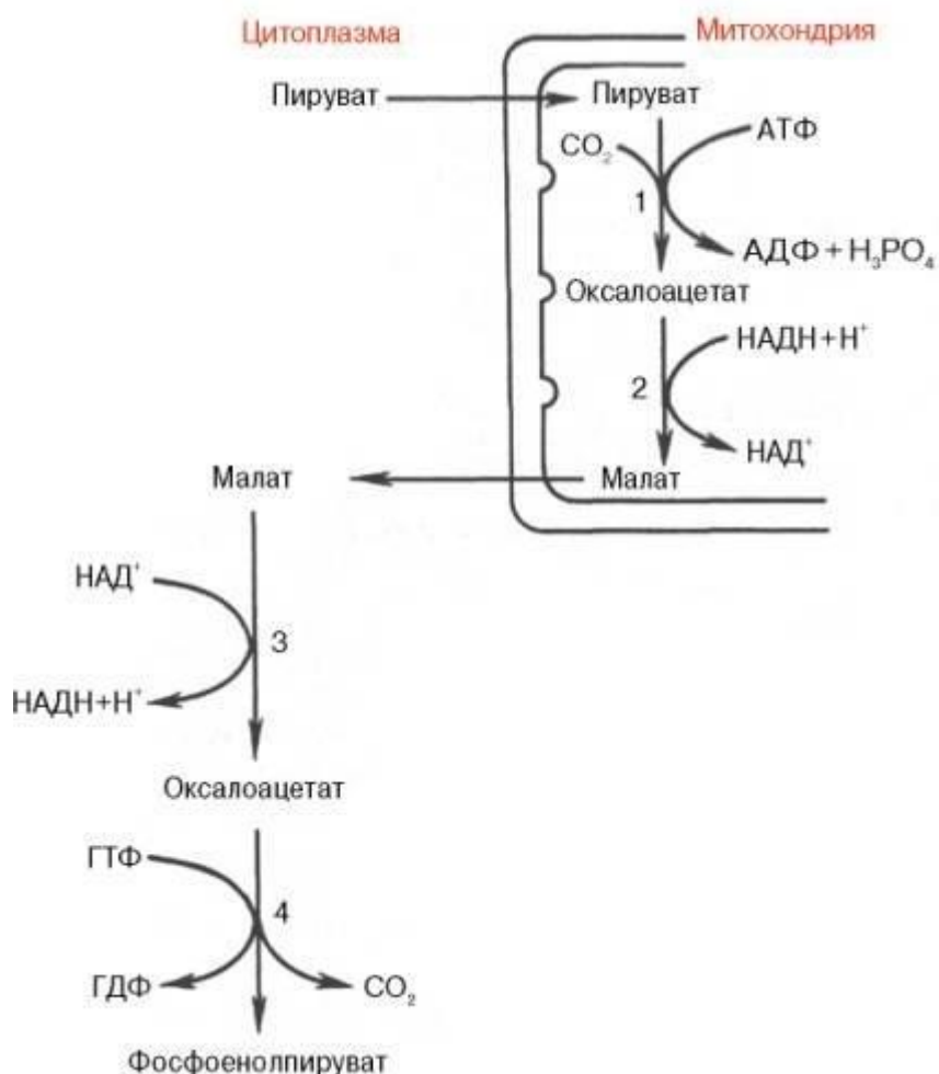
Рис. 10.6. Образование фосфоенол-пирувата из пирувата. 1 - пируваткарбоксилаза; 2 - малатде-гидрогеназа (митохондриальная); 3 - малатдегидрогеназа (цитоплазматическая); 4 - фосфоенолпируват-карбокси-киназа.
