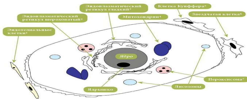
Рис.3 Структура гепатоцита
