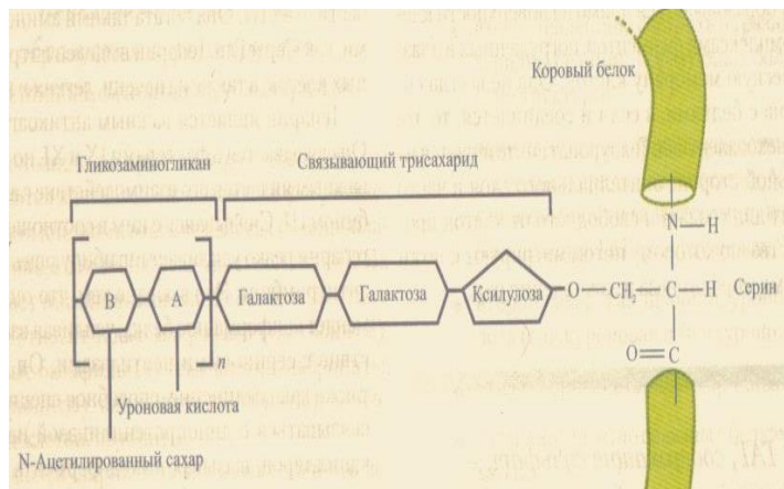
Рис.1. Связь линкерного участка ГАГ с серином коровьего белка.
